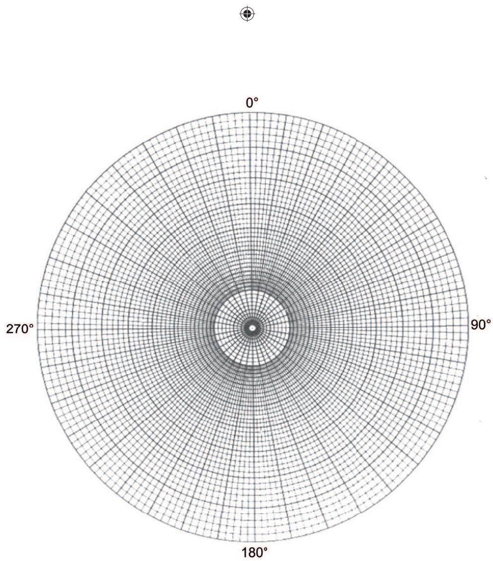
Příloha č. 1 Stereografická úhlojevná Wulfova síť v pólové projekci
